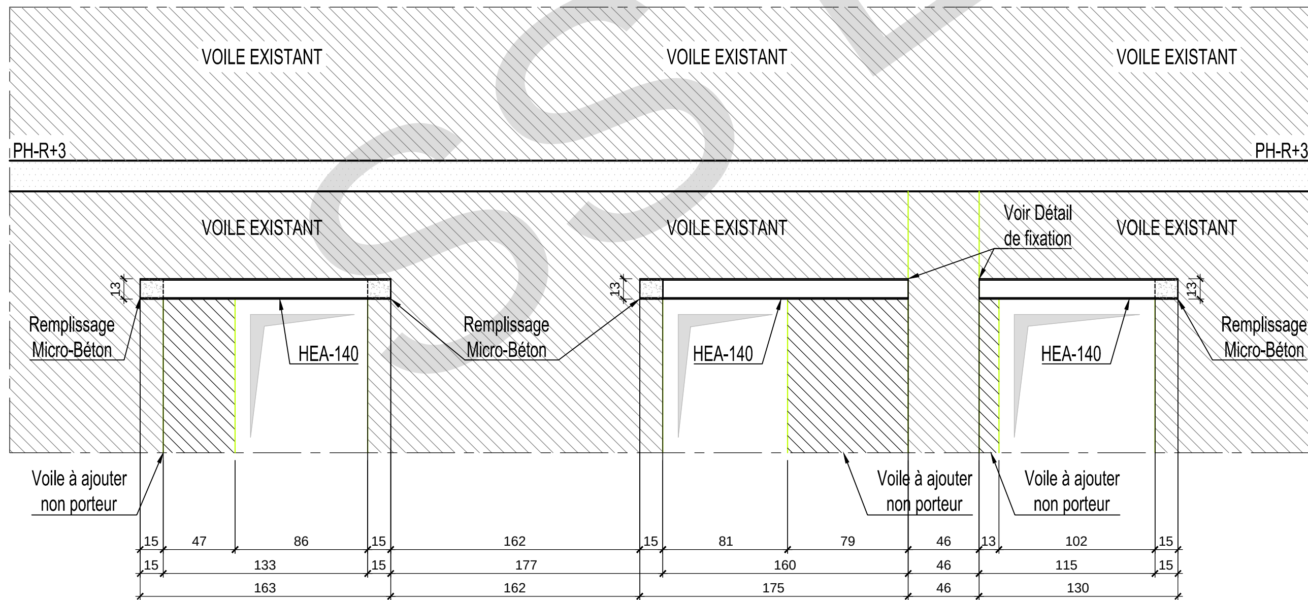
ELEVATION E1 Ech 1/25
