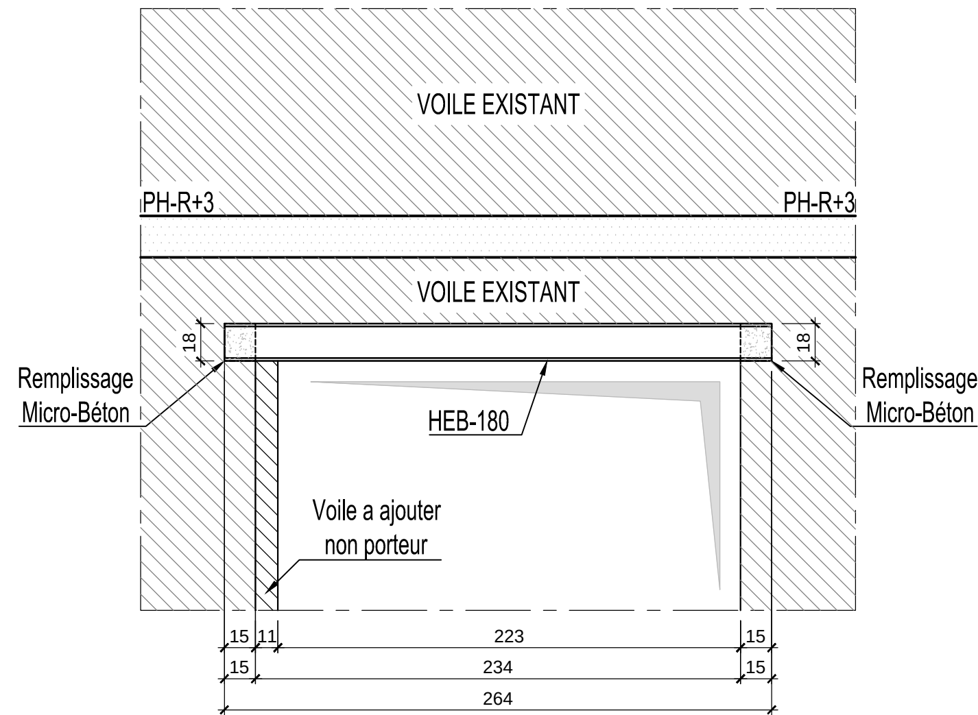
ELEVATION E2 Ech 1/25
